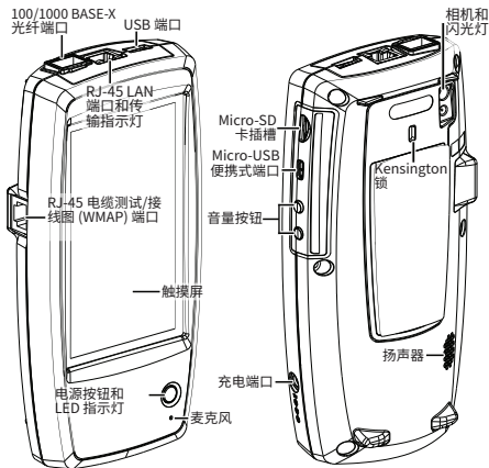
图 1: LinkRunner G2 物理特点
