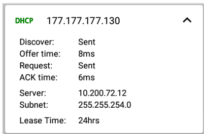
图 12: 扩展后的 DHCP 测试卡
