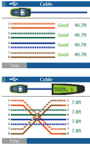
线缆布线验证
