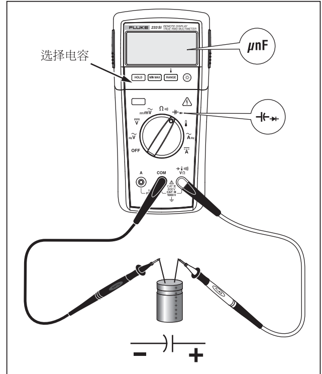
图 5. 电容测量
