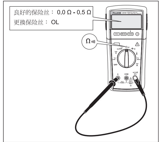
图 11. 保险丝测试
