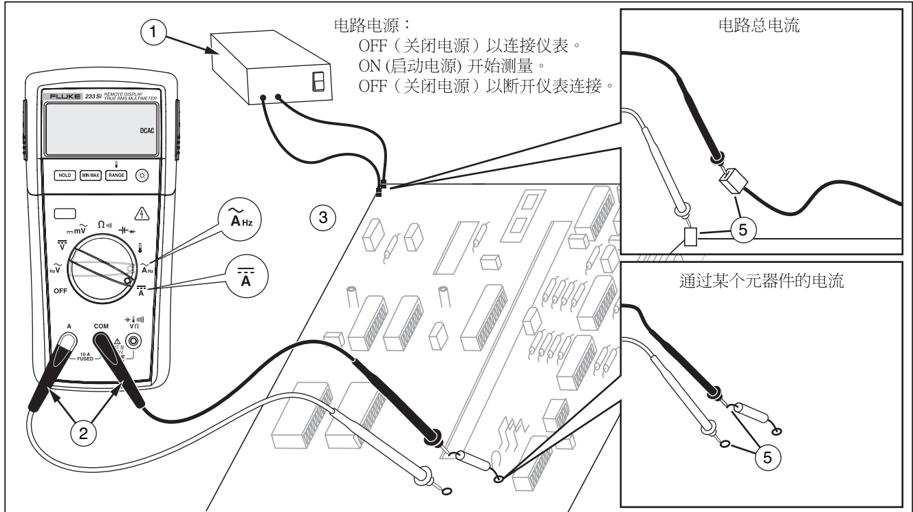
图 6. 电流测量
