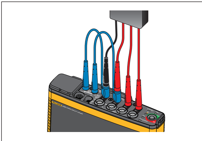
图示 7. 使用中性和仪器电源测量
