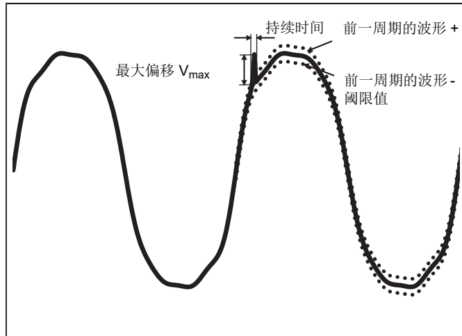
图示 14. 波形偏离
