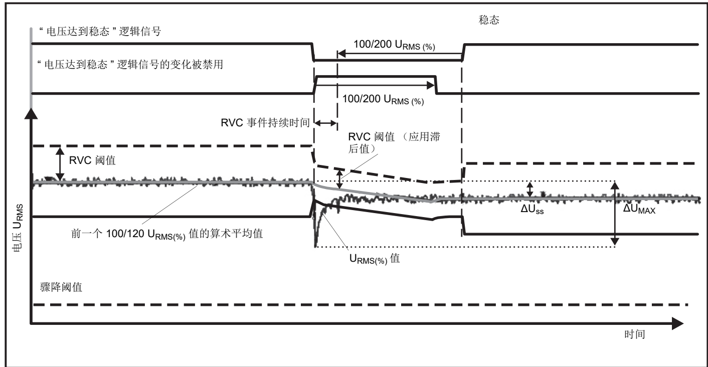
图示 13. 快速电压变化特性
