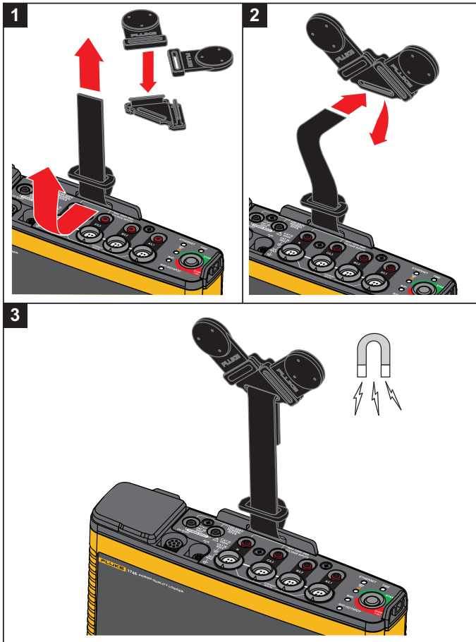
图示 2. 磁性挂带套件
