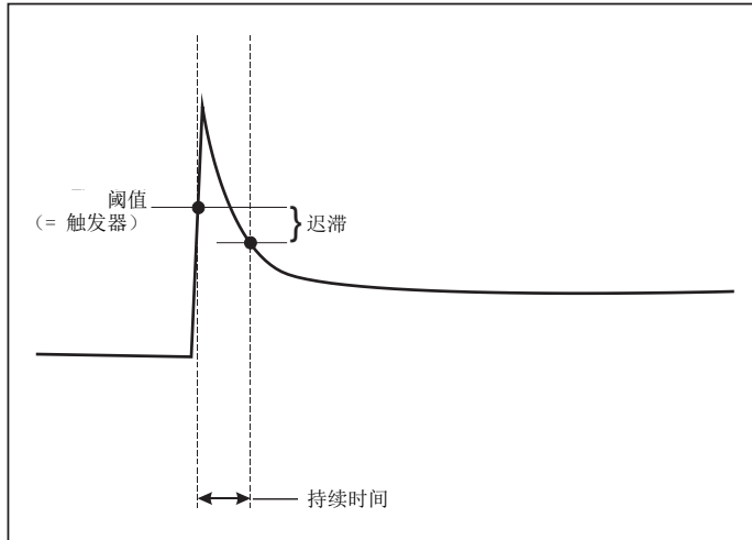
图示 15. 浪涌电流特性
