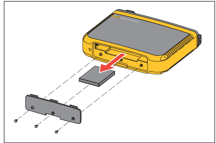
图示 16. 更换电池
