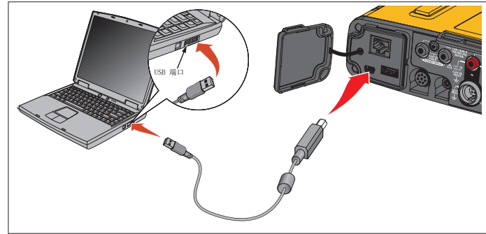
图示 9. Power Logger 至 PC 的连接
