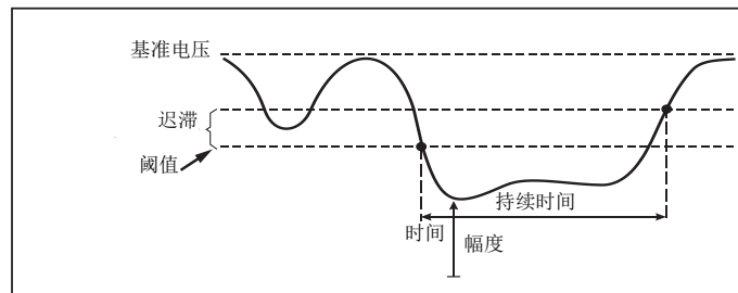
图示 10. 电压骤降的特征
