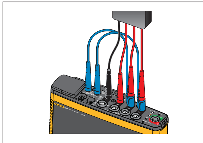
图示 8. 不使用中性电压和仪器电源测量
