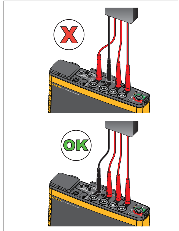
图示 6. 至 Logger 的测量连接
