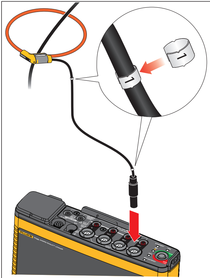
图示 4. 带有颜色编码的测试导线
