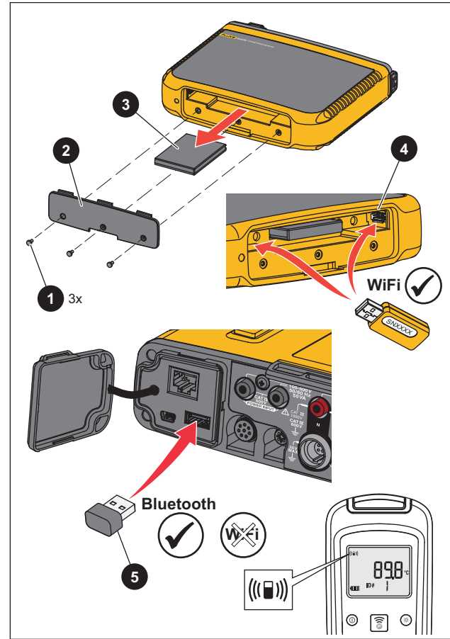
图示 1. 安装适配器
