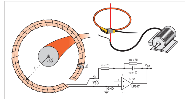
图示 3. R 线圈工作原理
