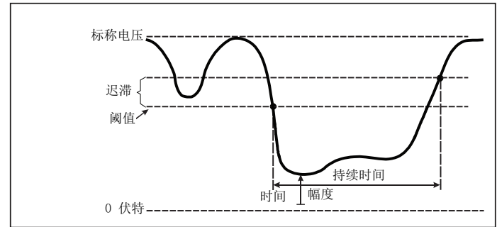
图示 12. 电压中断的特征
